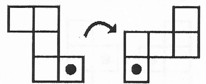
ROTATION
